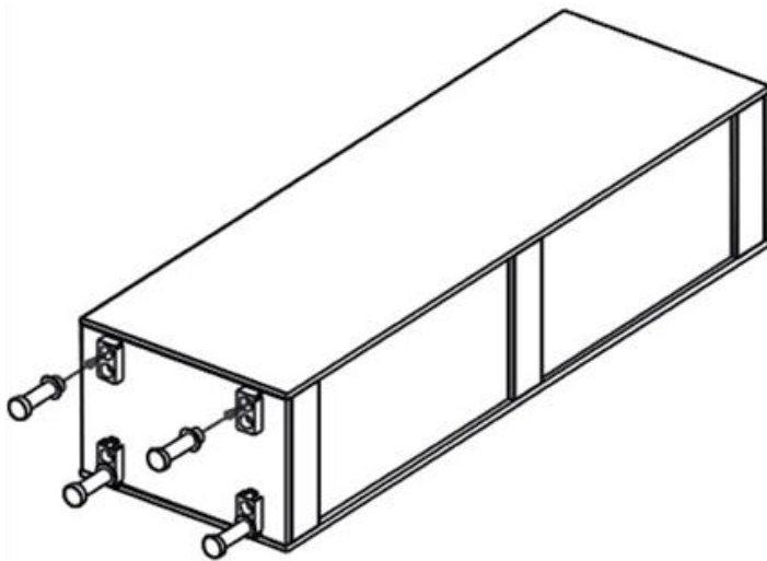
Sokkelijalkojen asennusperiaate
