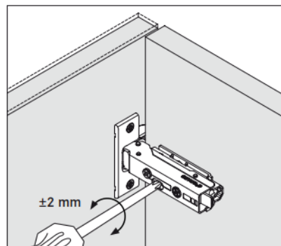
Korkeus-säätö
