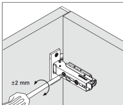
Sivuttais-säätö
