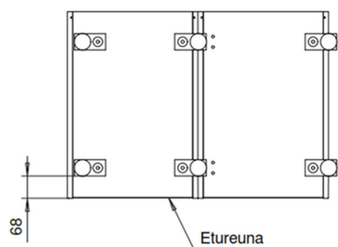
Sokkelijalkojen asennus
