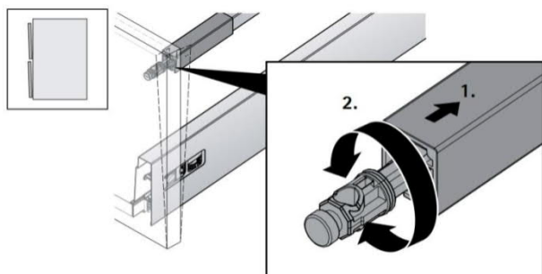
Laatikon syvyysäätö
