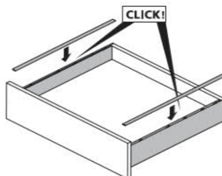
Laatikon peitelistat sivujen päälle
