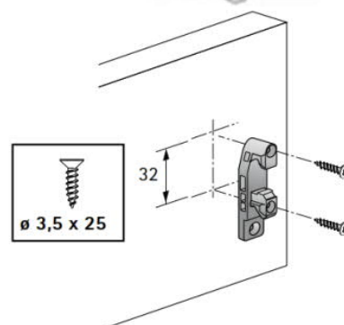
Ruuvikiinnitteinen etusarjan kiinnike
