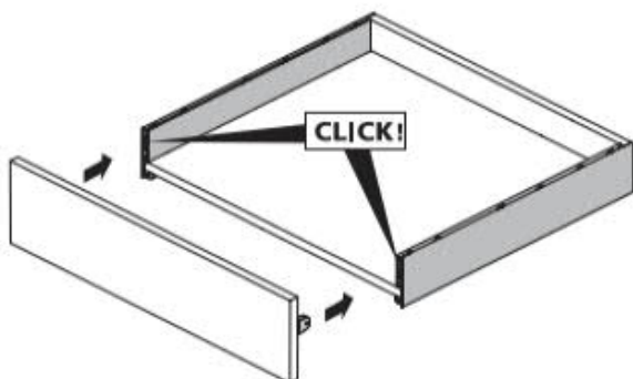
Etusarjan kiinnittäminen laatikkoon
