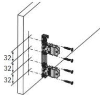
Ruuvikiinnitteinen etusarjan kiinnike, korkea
