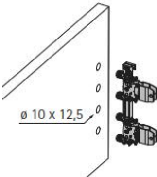
Etusarjan kiinnikkeen asennus, korkea
