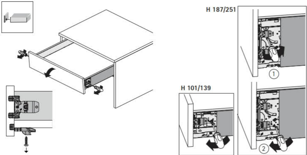
Etusarjan irrotus
