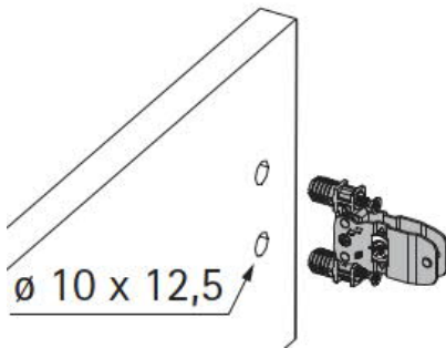
Etusarjan kiinnikkeen asennus, matala
