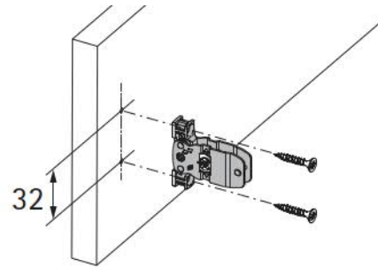
Ruuvikiinnitteinen etusarjan kiinnike, matala
