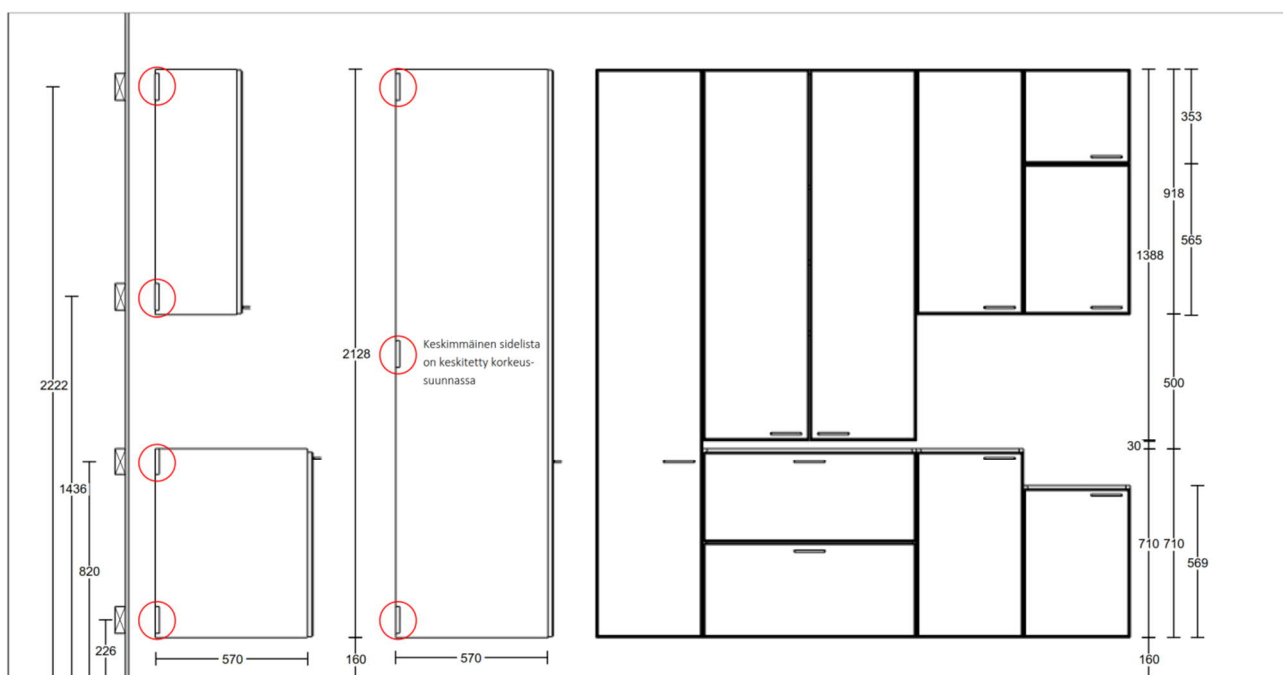
Korkeus 2288 normaali sokkelilla (160)
