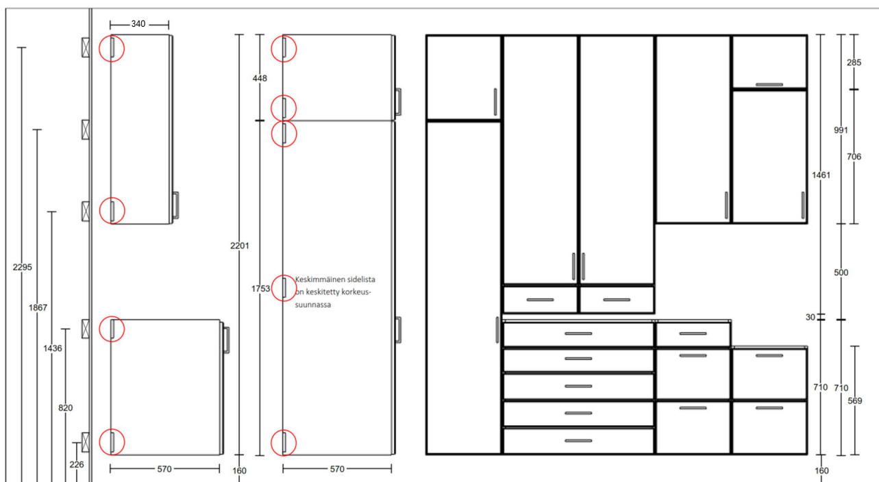
Korkeus 2361 normaali sokkelilla (160)
