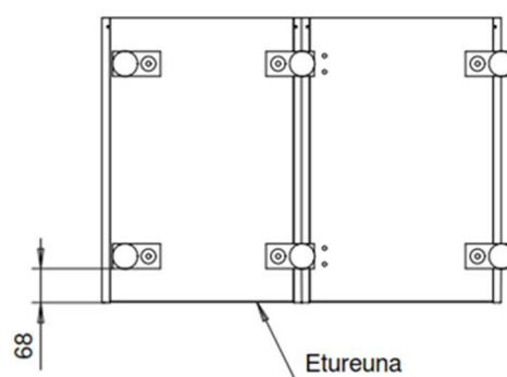
Sokkelijalkojen asennus
