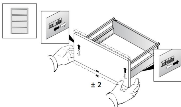
Laatikon korkeussäätö
