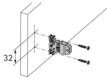
Ruuvikiinnitteinen etusarjan kiinnike, matala
