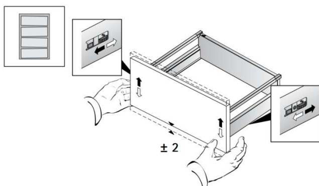
Laatikon korkeussäätö
