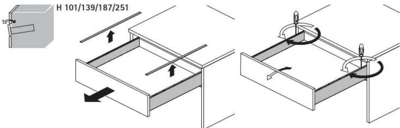
Laatikon syvyyssäätö
