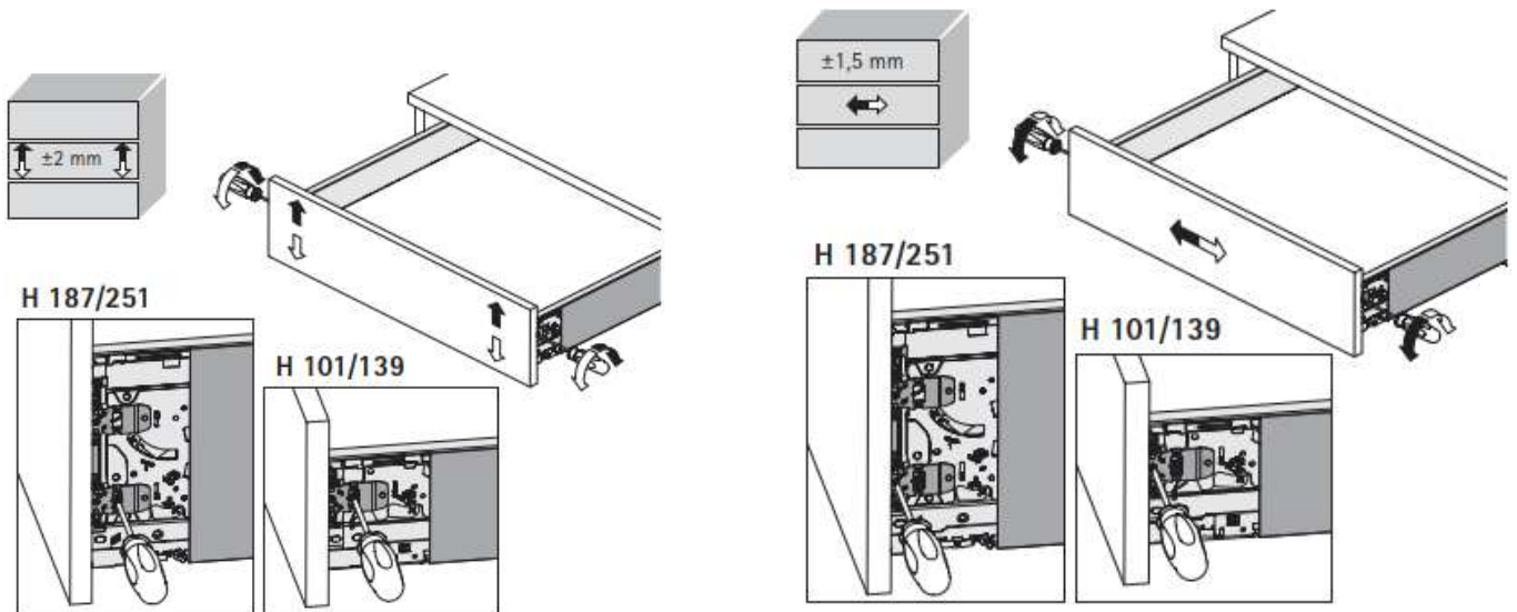
Laatikon korkeussäätö
