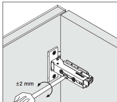
Korkeus-säätö
