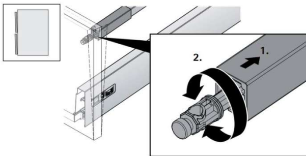
Laatikon syvyysäätö
