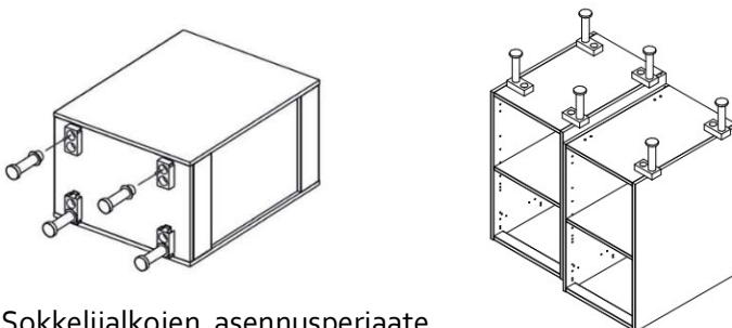
Sokkelijalkojen asennusperiaate
