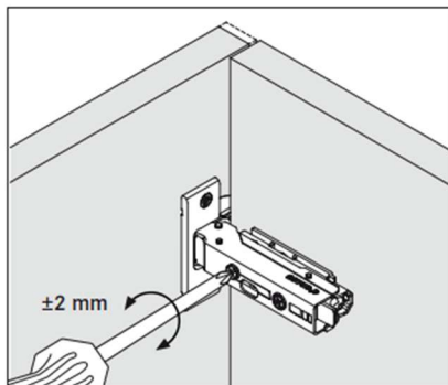
Sivuttais-säätö
