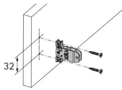
Ruuvikiinnitteinen etusarjan kiinnike, matala
