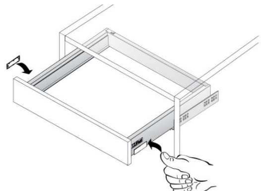
Säätöaukkojen peitelevyt
